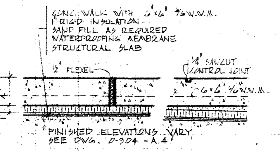
A. EXTERIOR CONZ. WALK
